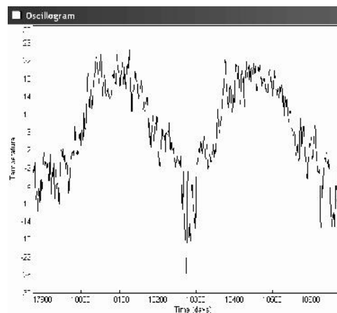
Рис.3. Пиковое похолодание (рис. 1), сглаженное тепловой инерционностью здания (постоянная времени – 1 сутки)
