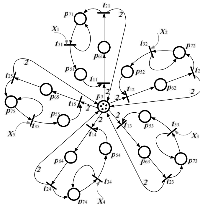
Рис. 2. Модель задачи об обедающих философях, представленная оценочной сетью Петри
