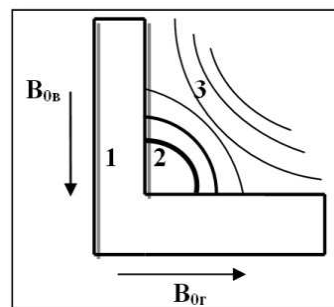
Рисунок 3 – Розподіл модуля вектора магнітної індукції у місцях примикання залізобетонних будівельних конструкцій: 1) залізобетонна конструкція; 2) зони підвищеного магнітного поля; 3) зони зниженого магнітного поля (рисунок не у масштабі)
