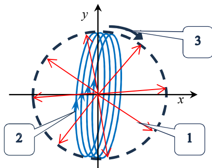
Рисунок 6 – Виникнення СПВ зі сферичною симетрією ліній 1 за рахунок колового вод'яного сєдвіча 2, який обертається навколо осі, що лежить в площині сєдвіча
