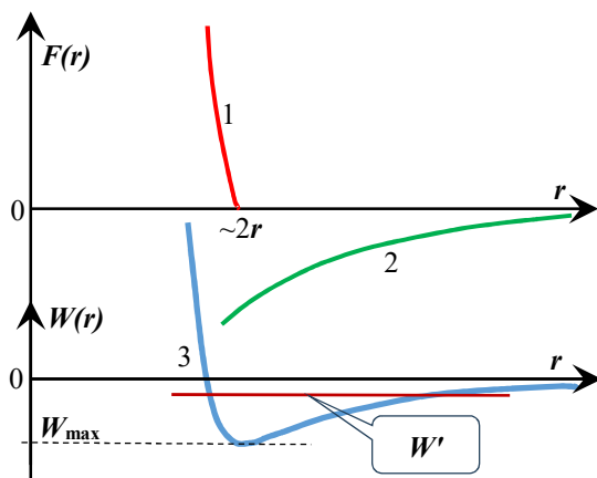
Рисунок 1 – Локальна корпускулярна взаємодія двох частинок: 1 – сили відштовхування, 2 – сили притягання, 3 – потенціальна енергія взаємодії
