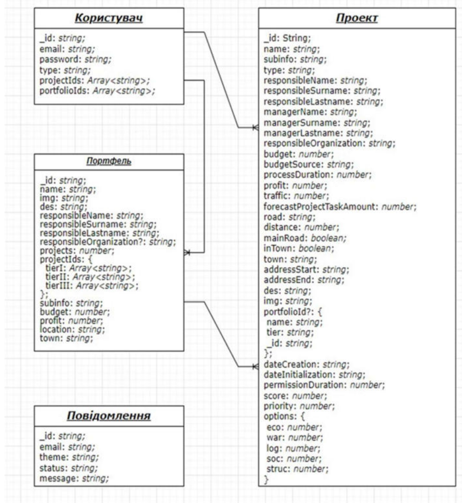
Рисунок 2 – Діаграма архітектури бази даних
